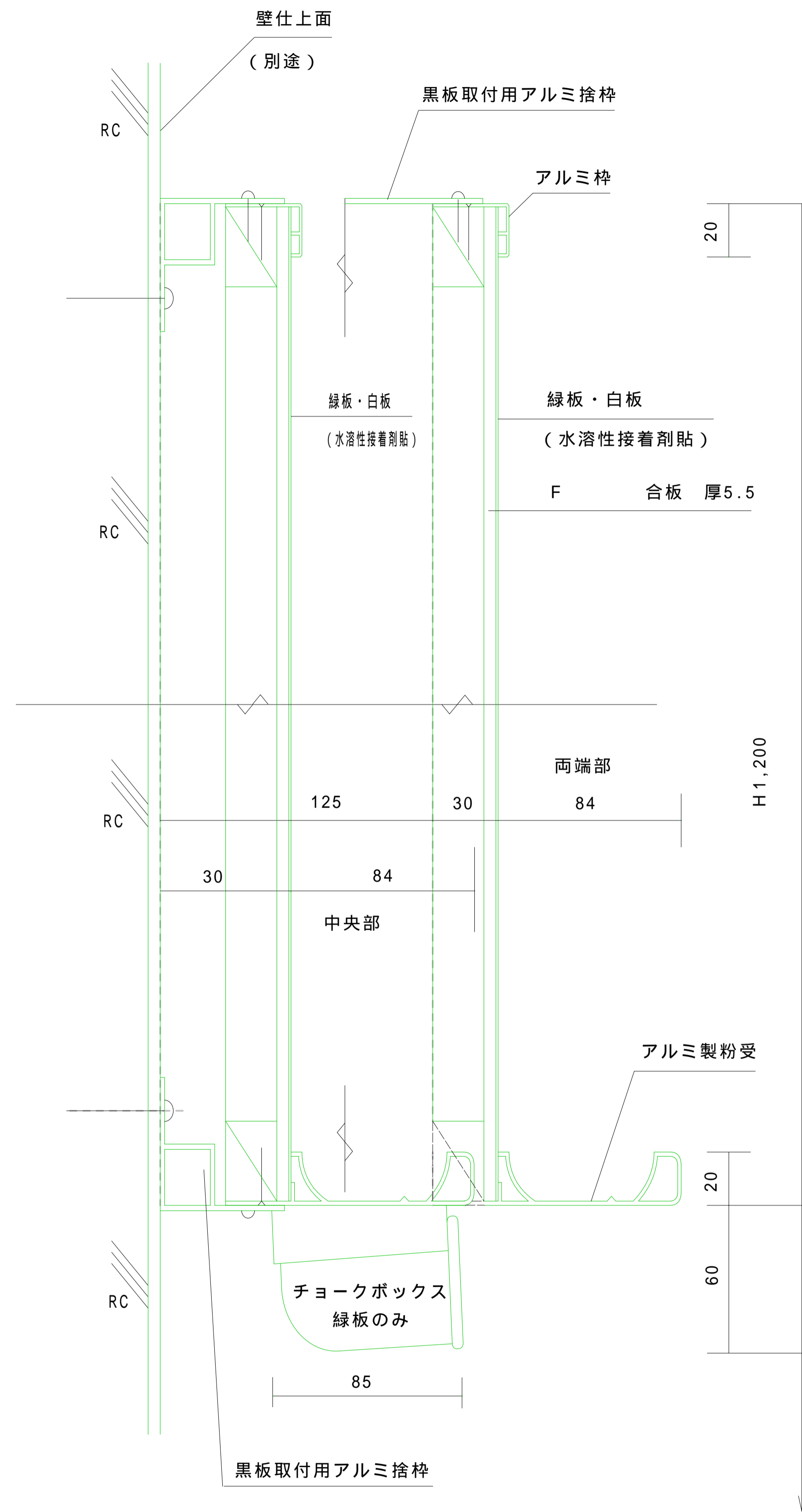
アルミ枠 曲面緑板・白板 捨枠式
