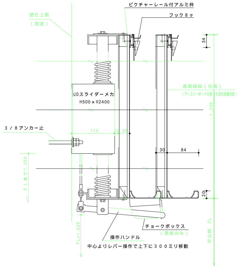
アルミ枠 UD式曲面スチール緑板(ホーロー白板) (アースリーボード仕様・水溶性接着剤貼) 断面図 1 / 3
