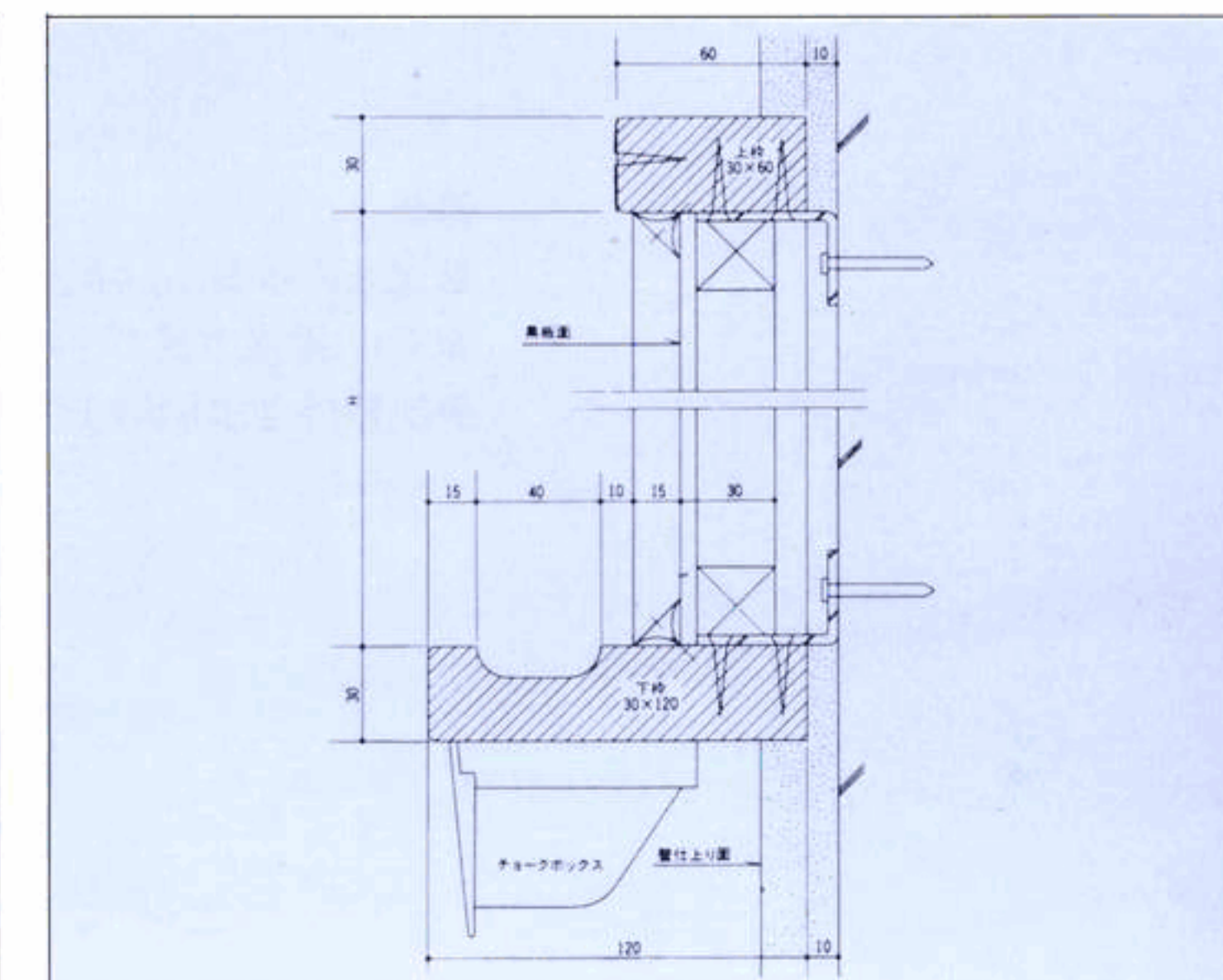
断面図
