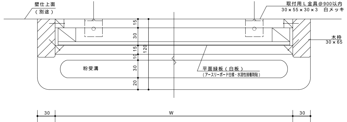
断面図 1 / 2
