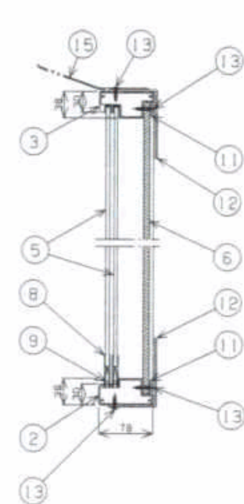
断面A-A
