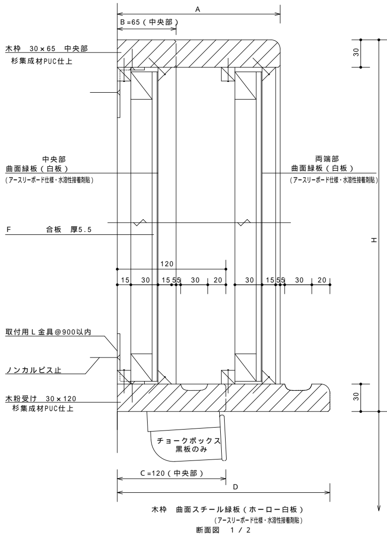
断面図 1 / 2
