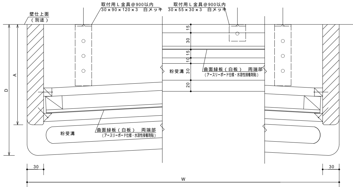
断面図 1 / 2
